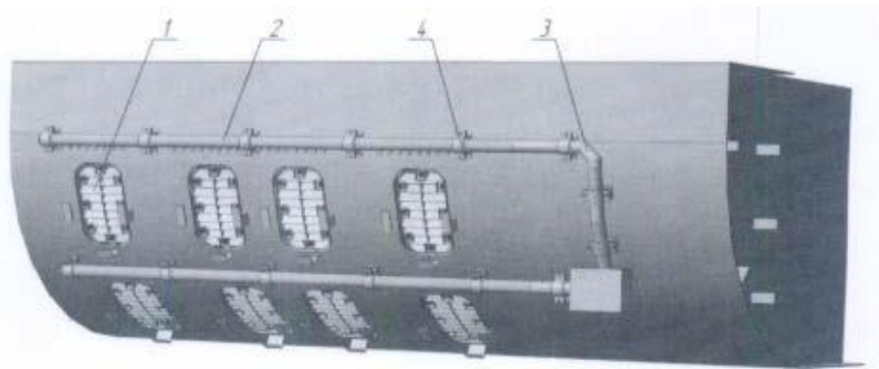
Рисунок 4.5 – РЗУ на водозаборных окнах кормовых кингстонных ящиков
