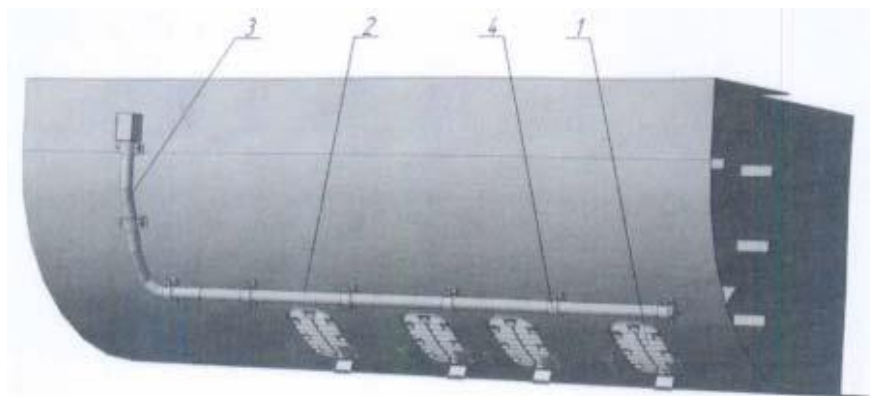
1 – кассета жалюзи; 2 – потокообразователь; 3 – стыковочный узел; 4 - замок
