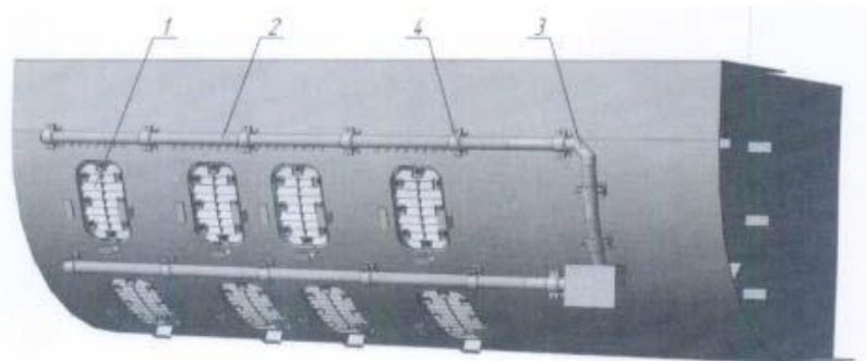
1 – кассета жалюзи; 2 – потокообразователь; 3 – стыковочный узел; 4 – замок Рисунок 4.5 – РЗУ на водозаборных окнах кормовых кингстонных ящиков
