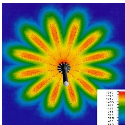
Рисунок 4.3 – Спектр температурных уровней пламени факела ( ^\circ\text{C} )
