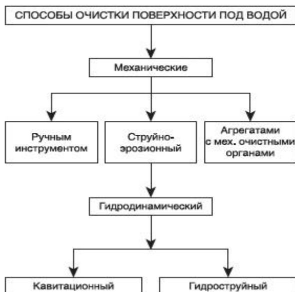
Рисунок 5.2 – Основные механические способы очистки поверхности от обрастания
